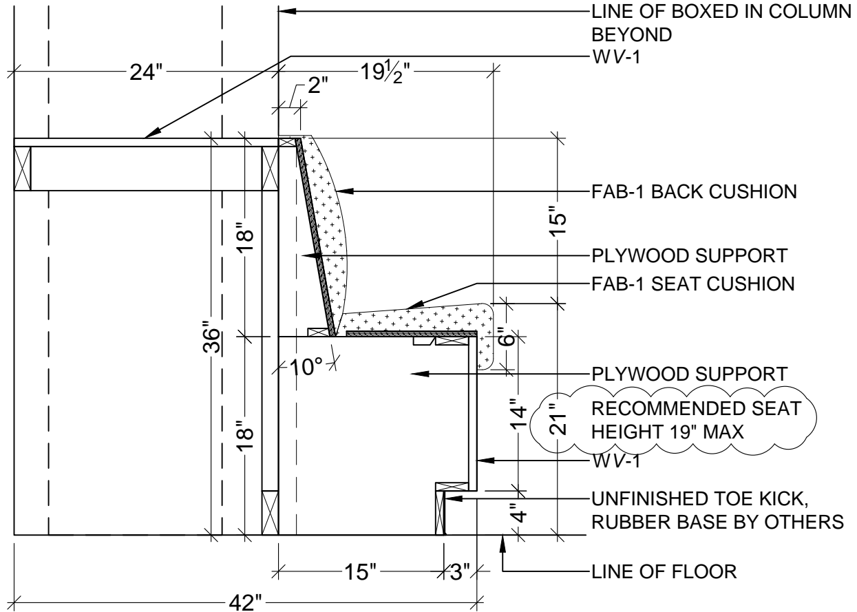
1 SECTION SCALE: 1" = 1'-0"
