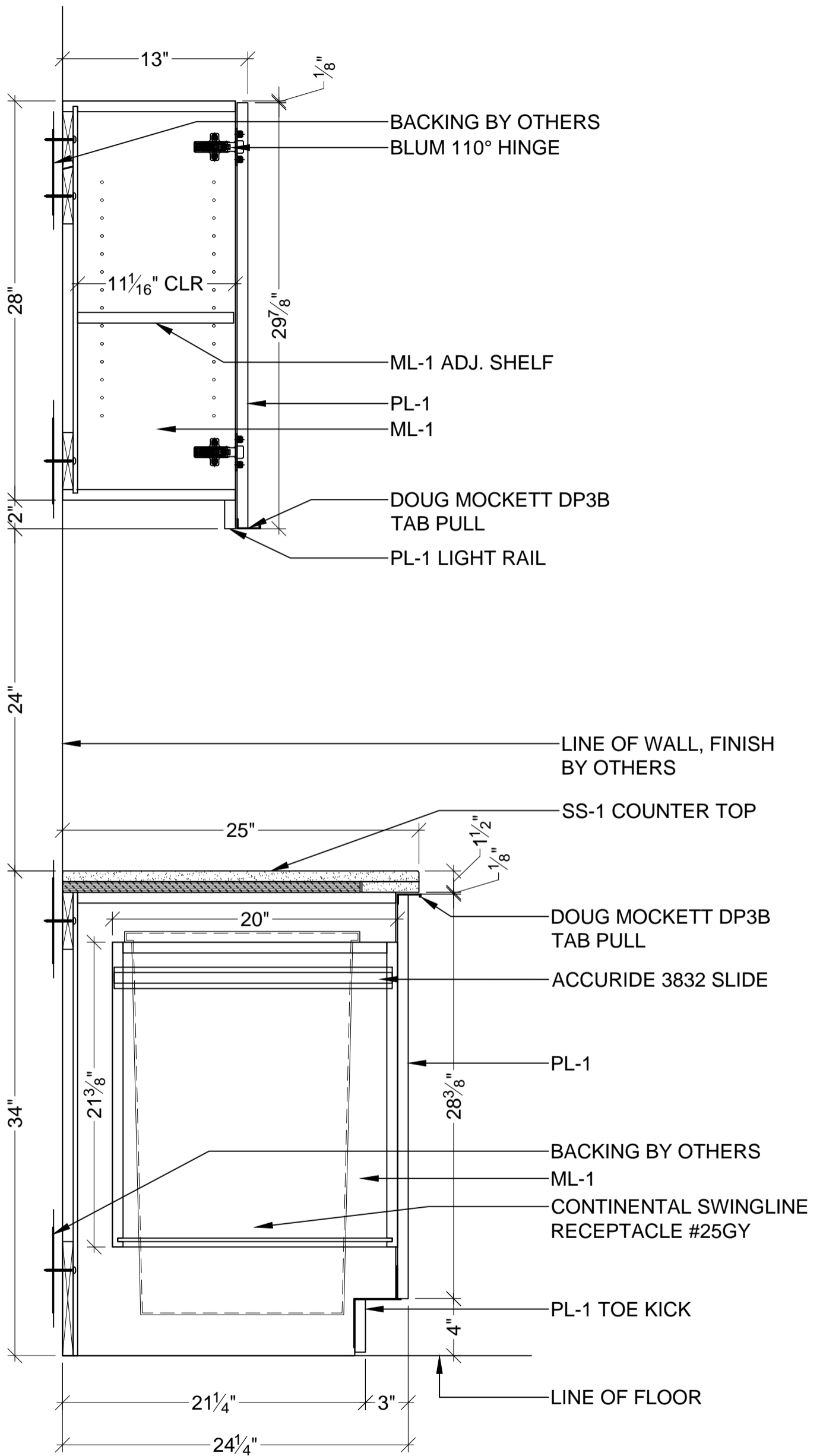
1 SECTION SCALE: 1 1/2" = 1'-0"
